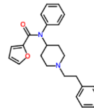
FURANYLFENTANYL
