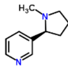
NICOTINE
